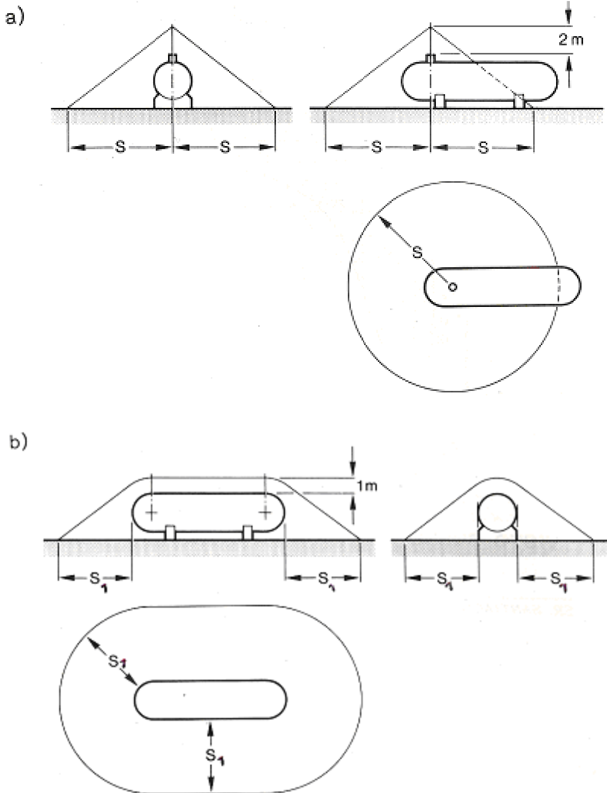
Figura 1.- Distancias mínimas de seguridad.
