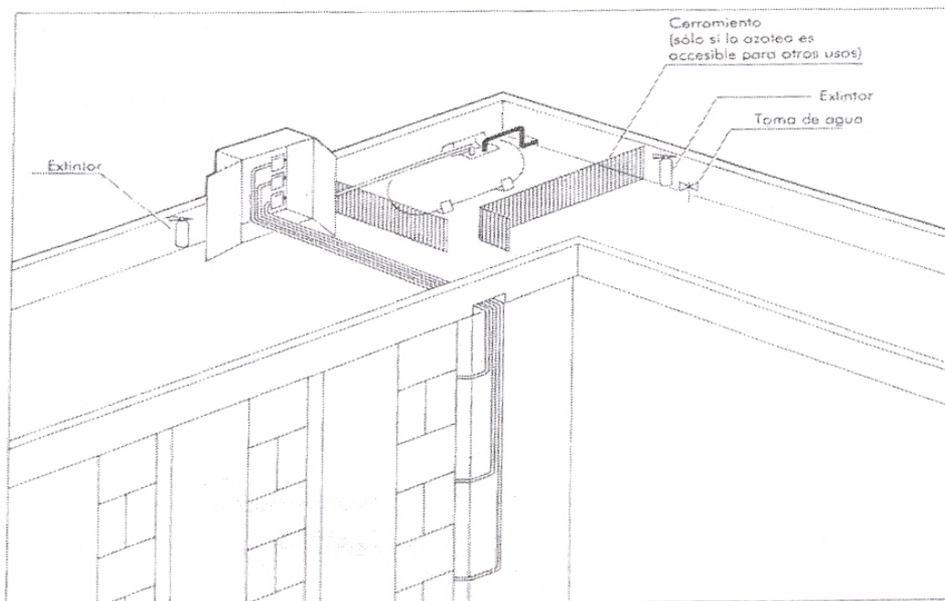
Figura 2.- Tanques en azoteas.
