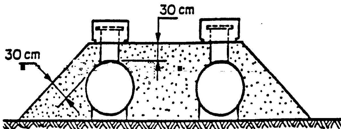
Figura 3.- Tanques en talud
