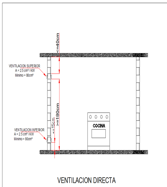
Figura 6. Ventilación directa.
