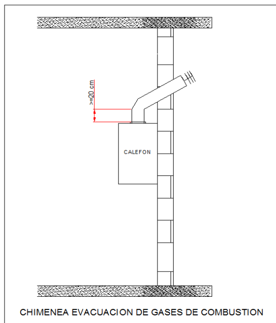
Figura 7. Chimenea de evacuación de gases.
