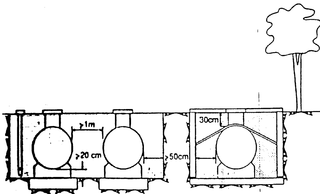
Figura 4.- Tanques enterrados.
